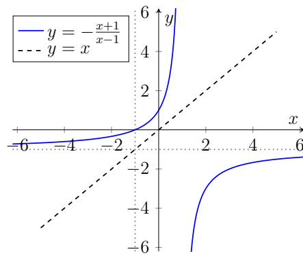
Graph der Funktion f^{-1}
